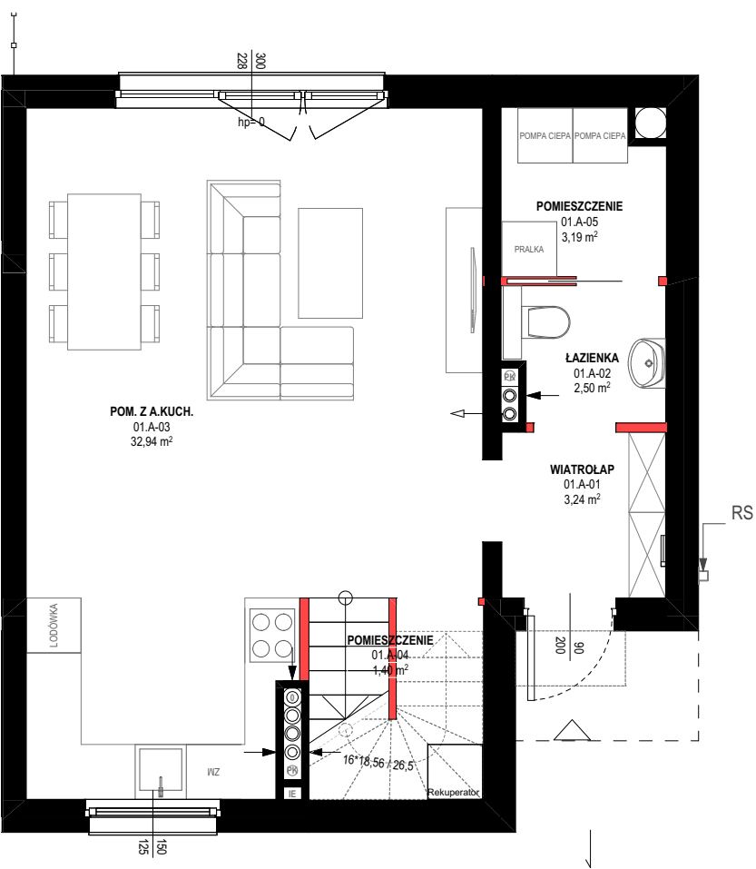
RZUT PARTERU
