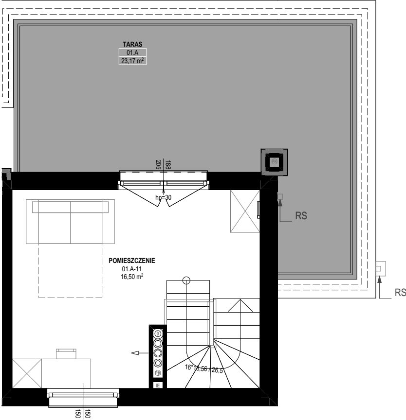
RZUT 2 PIĘTRA
